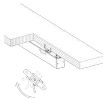
Deckenhalterung 2 Stk Art.Nr. 457060 9,50 €
